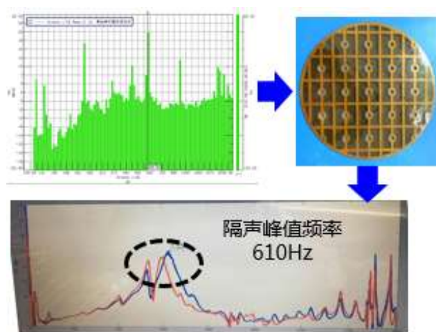
Figure 1 声学超材料的隔声量测量
