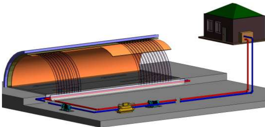
图 2 地铁源热泵基本构成
