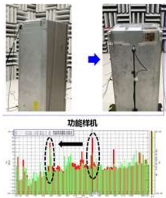
Figure 2 冰箱噪声测量， 红色，使用声学超材料前，绿色，使用声学超材料后
