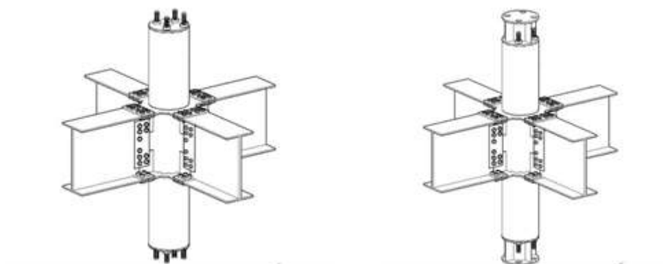
图 1 装配式自恢复圆形钢管混凝土组合节点
