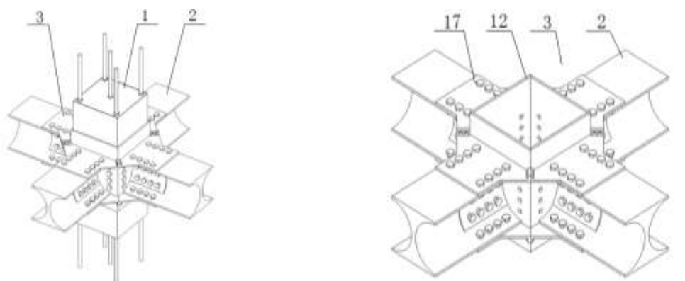
图 11 装配式限位增强钢木磨砂套筒组合节点
