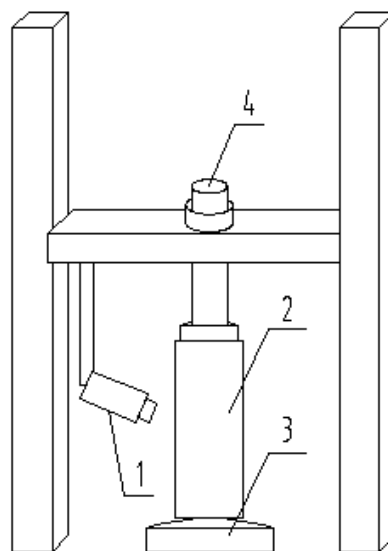
图 2. 实验装置的主体结构原理示意图
