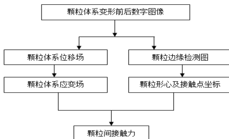
图 1. 工作原理流程示意框图
