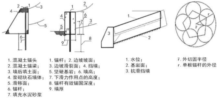
图5 滑坡重力式锚杆图6 滑坡悬臂式锚杆图7 滑坡抗滑挡墙示意图图8 滑坡锚杆束加固
