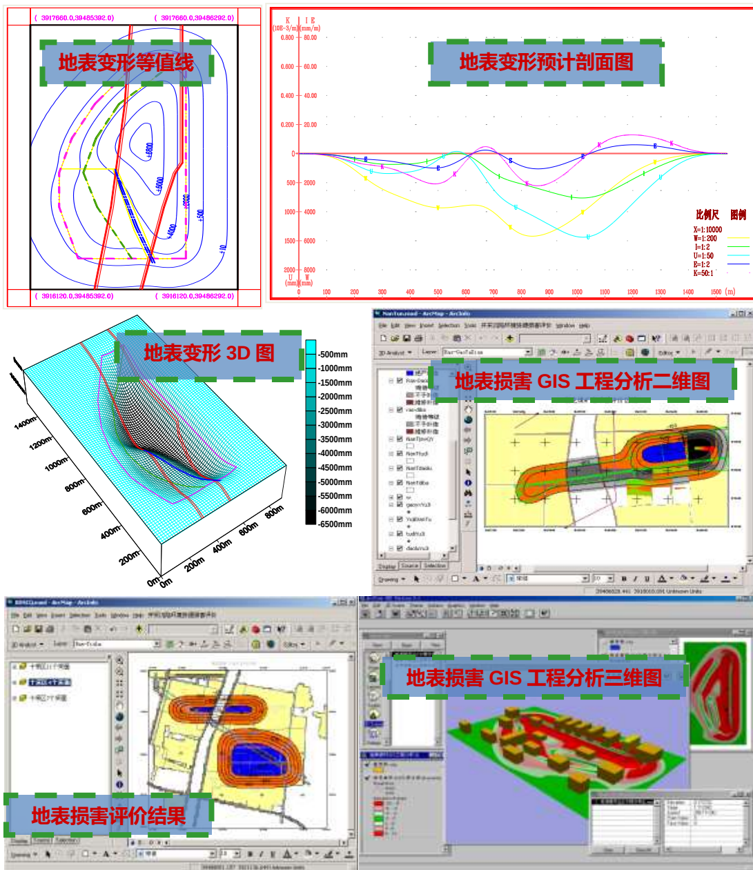
开采沉陷预计及地表损害结果图形输出
