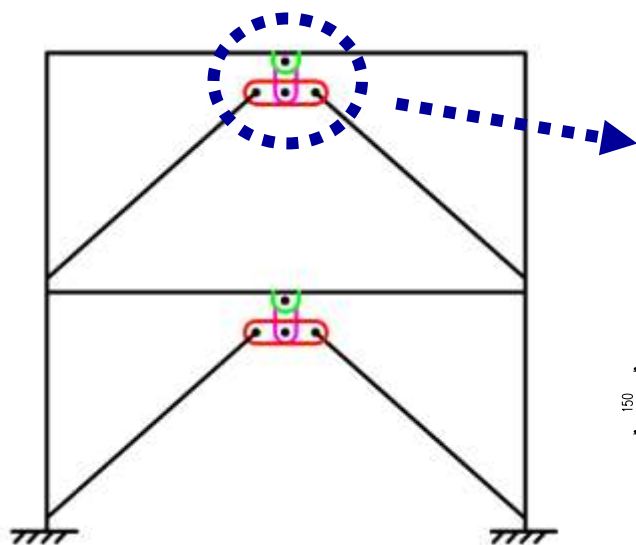
摩擦阻尼器在钢框架结构中的应用
