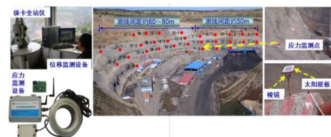
滑动力-位移耦合滑坡综合监测装备
