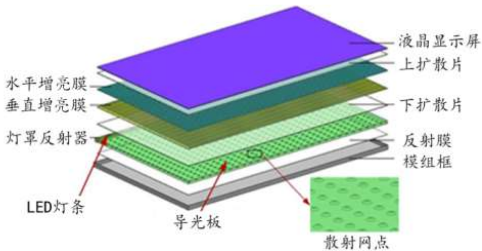
背光源模组示意图
