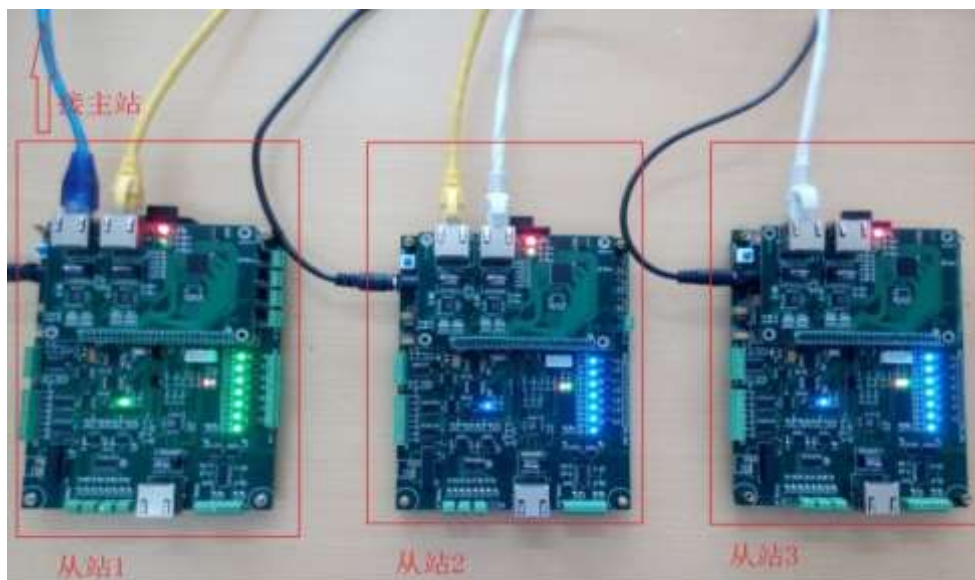
基于 EtherCAT 总线的分布式测控系统
