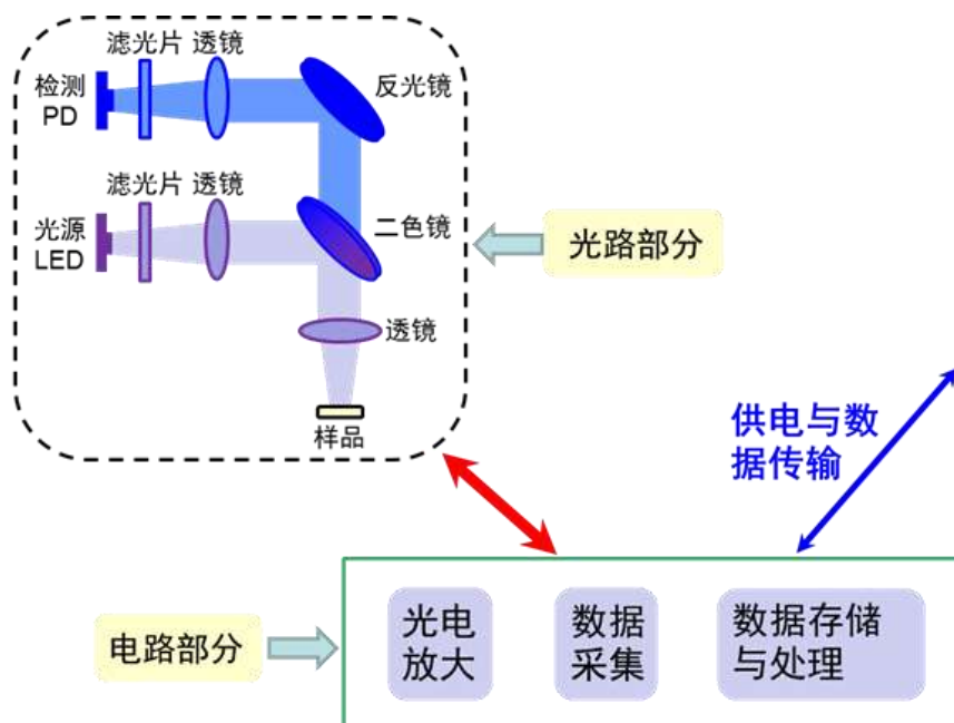
图 2 荧光传感器工作原理图
