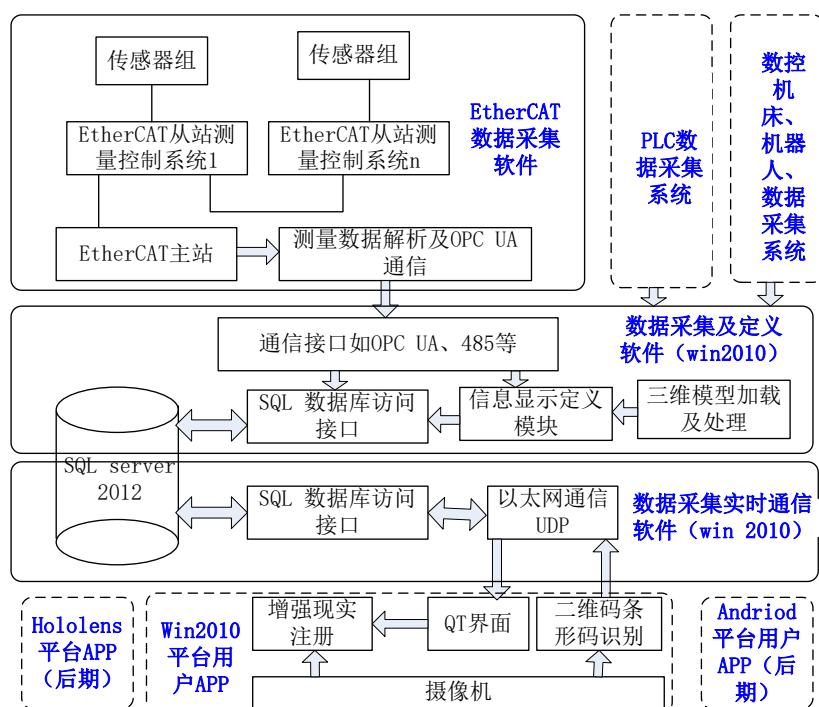
增强现实数字化显示平台架构图
