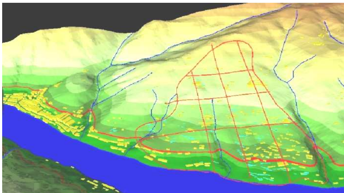
三维可视化边坡稳定性综合分析 (3D Slope Pro SPRM- II)
