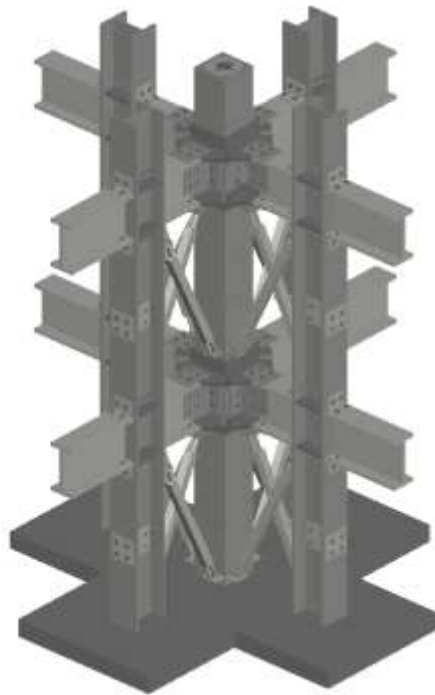
可拼接分割板的多层耗能式钢管混凝土组合柱
